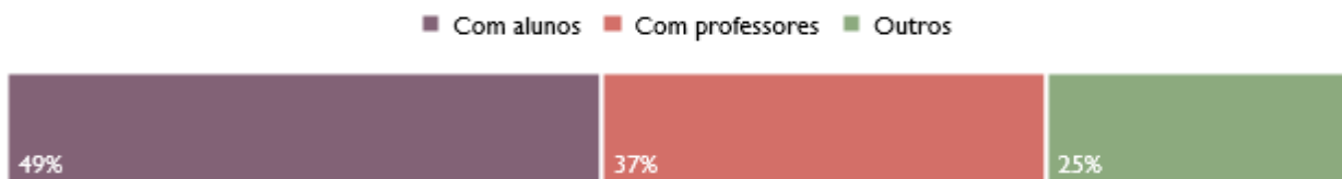
Avaliação Informal (116)
