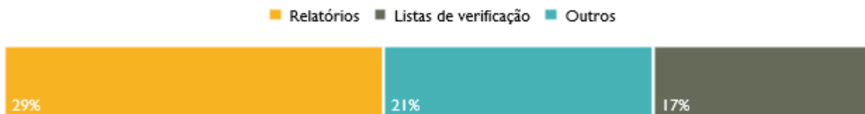
Avaliação Formal (76)
